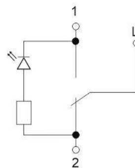
выключатель одноклавиш-ный проходной с индикацией
