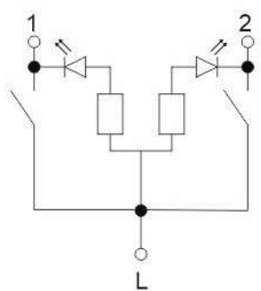
выключатель двухклавиш-ный с индикацией
