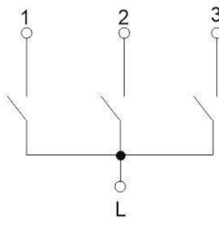
выключатель трехкла-вишный
