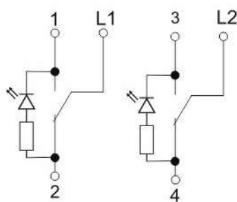
выключатель двухклавиш-ный проходной с индикацией
