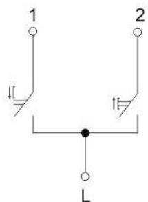
выключатель жалюзи
