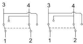
выключатель двухкла-вишный
