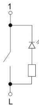
выключатель одноклавиш-ный с индикацией
