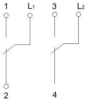
выключатель двухклавиш-ный проходной
