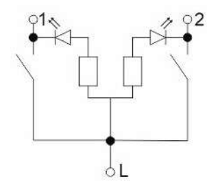
выключатель двухклавишный с индикацией
