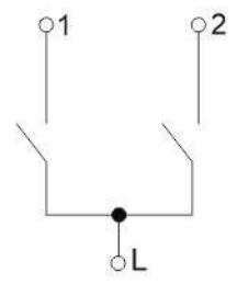
выключатель двухклавишный
