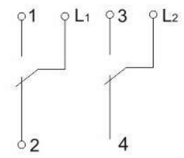
выключатель двухклавишный проходной
