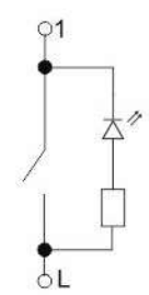
выключатель одноклавишный с индикацией
