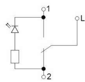
выключатель одноклавишный проходной с индикацией
