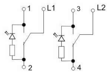
выключатель двухклавишный проходной с индикацией
