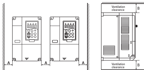
Рис. 4-1 Монтажная схема
