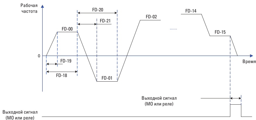
Схема работы простого ПЛК
