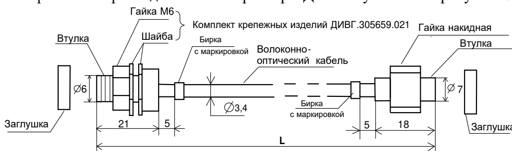
Рисунок 1 - Габаритные и присоединительные размеры Датчика
