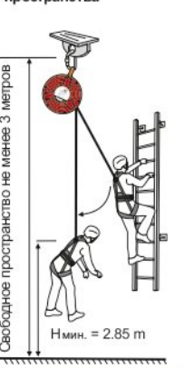
Рис. 11. Вытягивание и втягивание троса
