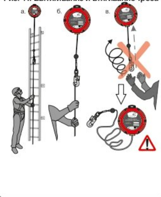
Рис. 11. Вытягивание и втягивание троса
