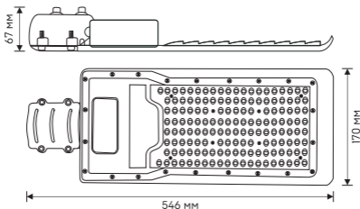
Рис. 4 - Габаритные размеры светильника ДКУ-9004-Ш
