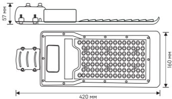
Рис. 3 - Габаритные размеры светильника ДКУ-9003-Ш
