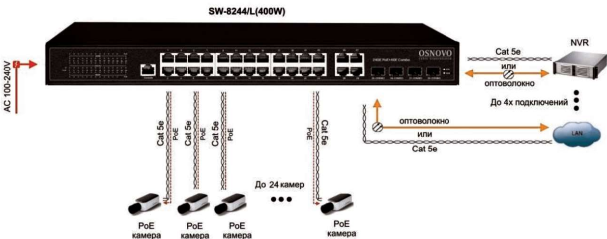
Рис.8 Типовая схема подключения коммутатора SW-8244/L(400W)
