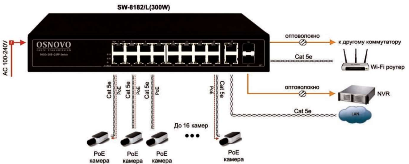
Рис.7 Типовая схема подключения коммутатора SW-8182/L(300W)
