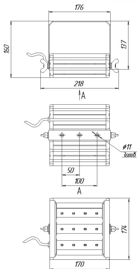
Светильник УСС 18 с 2Ех маркировкой потолочное крепление
