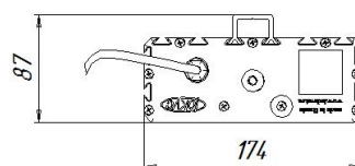
Светильник УСС 18 с 2Ех маркировкой потолочное крепление
