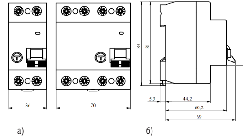
а) Рисунок Б.1 Габаритные, установочные и присоединительные размеры ВДТ
