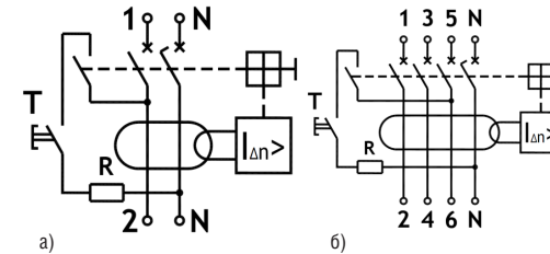
Рисунок В.1 Принципиальные электрические схемы ВДТ
