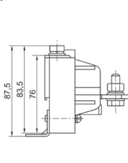
Реле для индивидуальной установки
