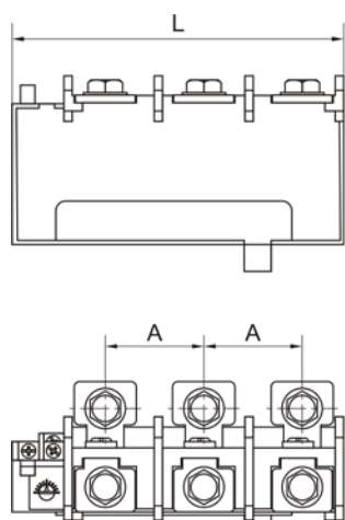
Рисунок 2. Габаритные и установочные размеры реле серии PTT-325, PTT-326, PTT-327
