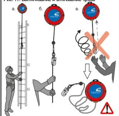
Рис. 11. Вытягивание и втягивание троса
