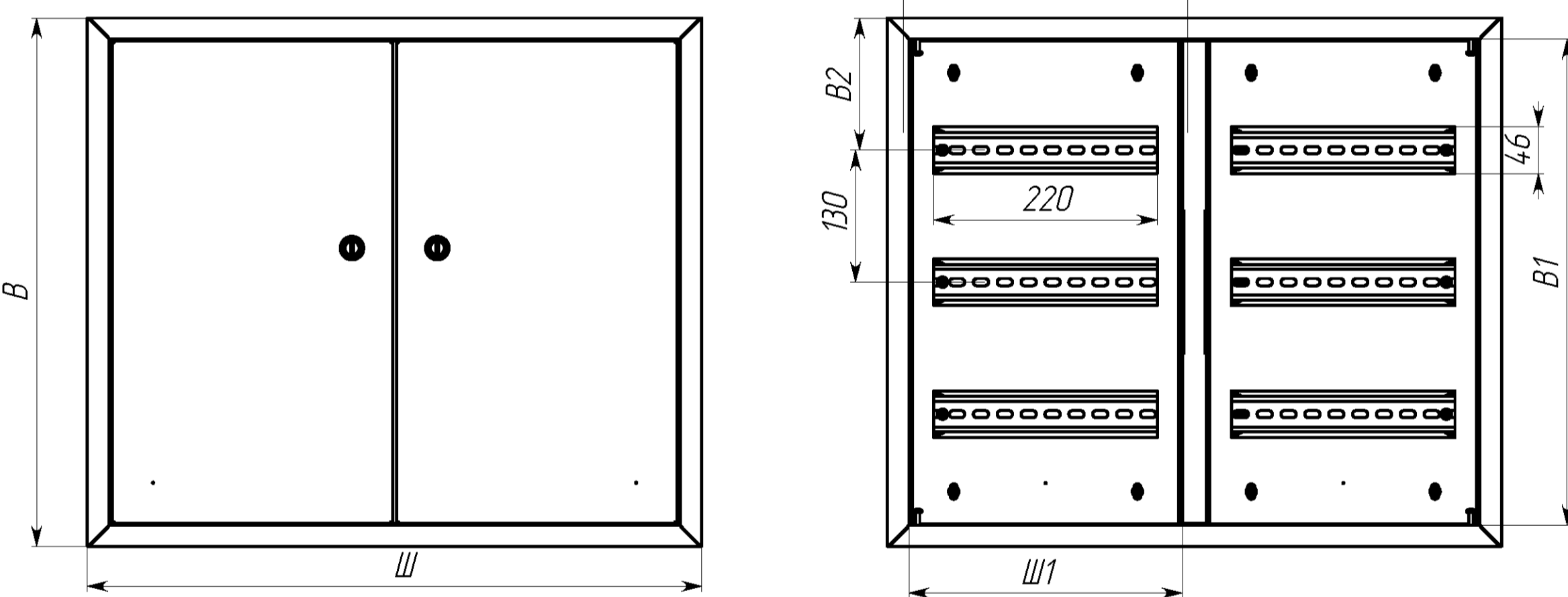
Вид спереди
