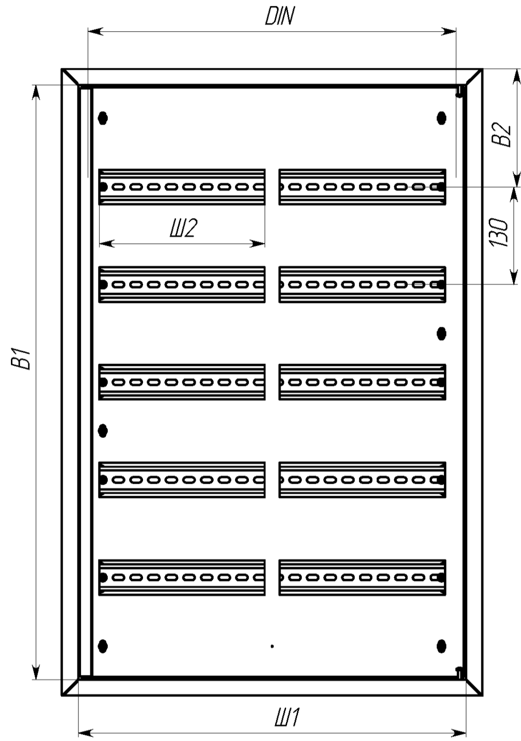
Вид без дверей
