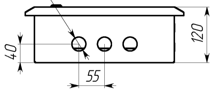
\phi 30 п отв.
