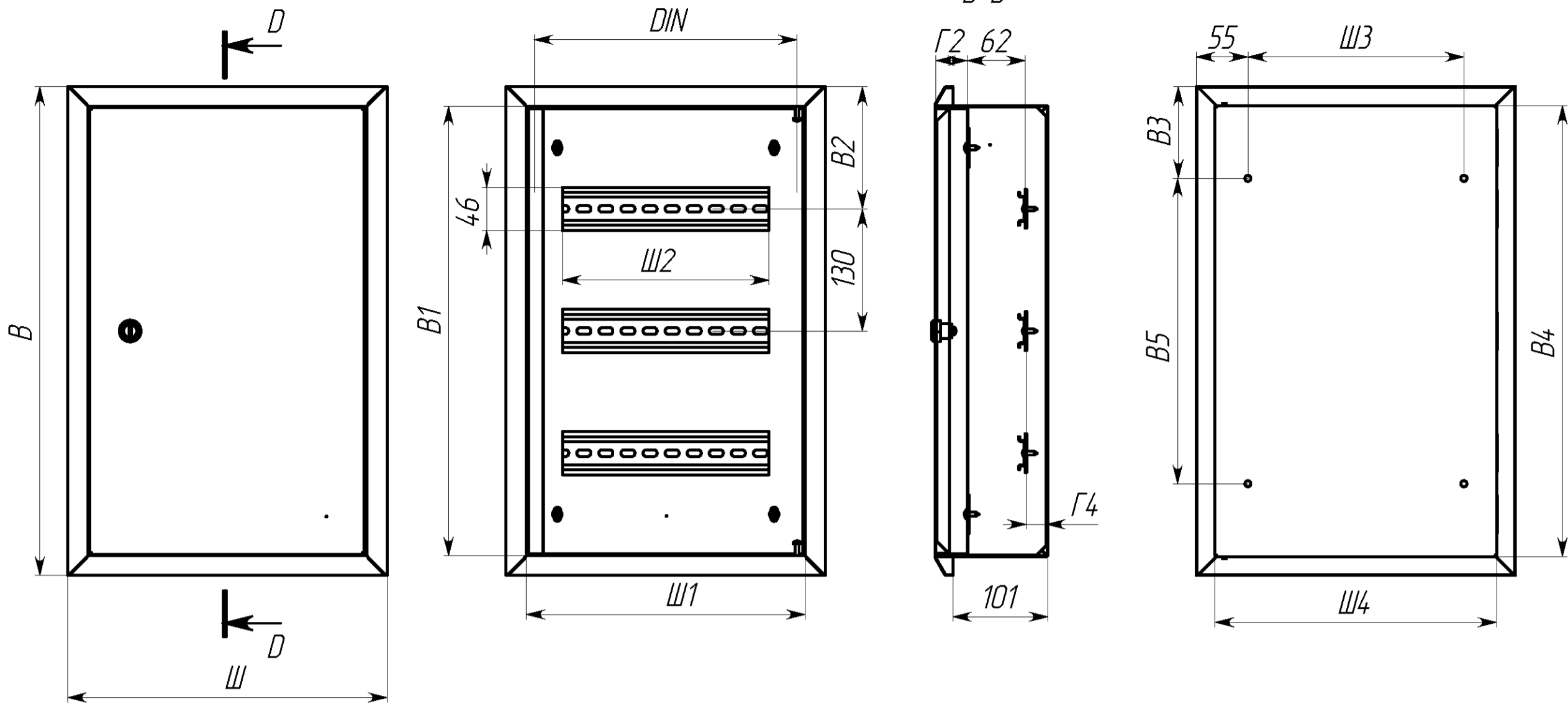
Вид без двери
