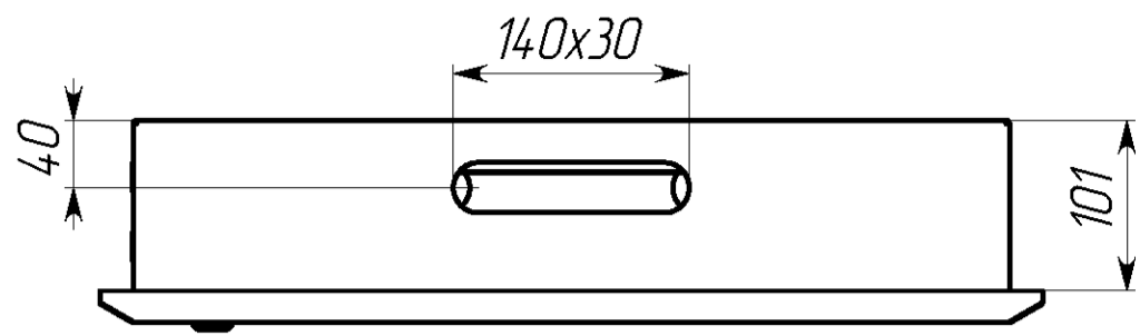
Вид сверху
