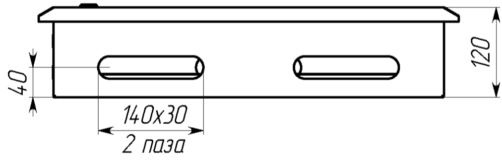
Вид снизу
