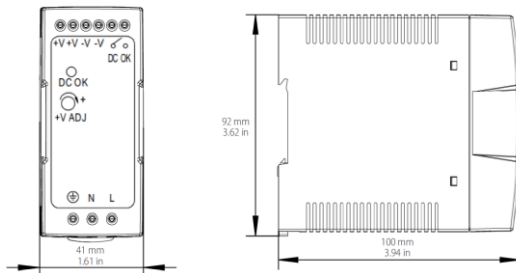
Рисунок 2. Внешний вид и обозначение клемм SMARTWATT PSE DRS 2430, 2440, 2460.
