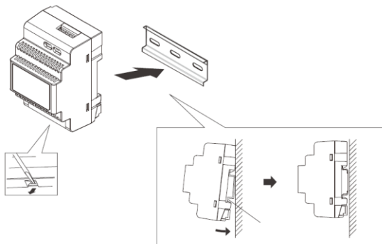
Рисунок 10. Установка блока питания на DIN-рейку.
