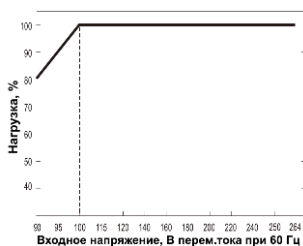
Рисунок 12. График зависимости нагрузочной способности блока питания от входного напряжения.
