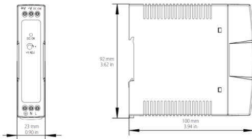
Рисунок 1. Внешний вид и обозначение клемм SMARTWATT PSE DRS 2420.
