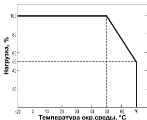
Рисунок 11. График зависимости нагрузочной способности блока питания от температуры окружающей среды.
