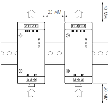
Рисунок 9. Размещение блока питания.
