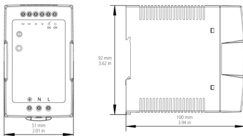
Рисунок 3. Внешний вид и обозначение клемм SMARTWATT PSE DRS 24100.
