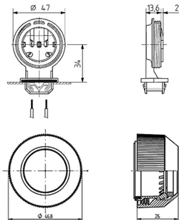
Патрон (ламподержатель) герметичный G13 для люминесцентных ламп T8, одиночный IP67 (водо- и пылезащищенный) с прижимной муфтой под лампу Ø 26мм в сборе (крепление на защелки), серый
