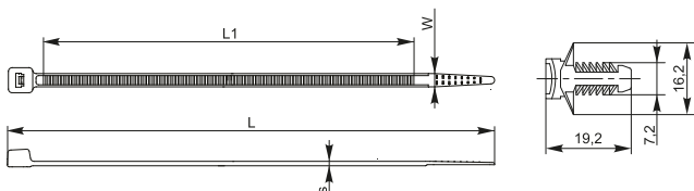
Рисунок / Сурет 9 – Размеры хомутов для вентиляции / Желдетуге арналған қамыттардың өлшемдері
