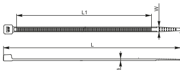
Рисунок / Сурет 1 – Размеры стандартных кабельных стяжек / Стандартты кабель тартпаларының өлшемдері
