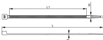
Рисунок / Сурет 7 – Размеры съёмных хомутов / Алмалы-салмалы қамыттардың өлшемдері
