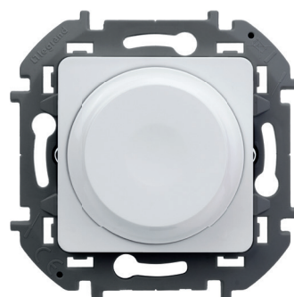
СВЕТОРЕГУЛЯТОР ПОВОРОТНО- НАЖИМНОЙ УНИВЕРСАЛЬНЫЙ (5-75 Вт для LED-ламп, 5-300 Вт для ламп накаливания)
