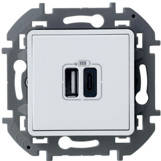
USB-РОЗЕТКА ТИП А / ТИП С 3000 МА - 5 В
