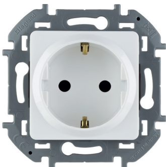
РОЗЕТКА 2К+3 СО ШТОРКАМИ 16 А - 250 В ~
