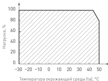
Рис. 2. Максимальная допустимая нагрузка, % от мощности источника
