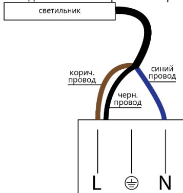
Рис. 2 Схема подключения
