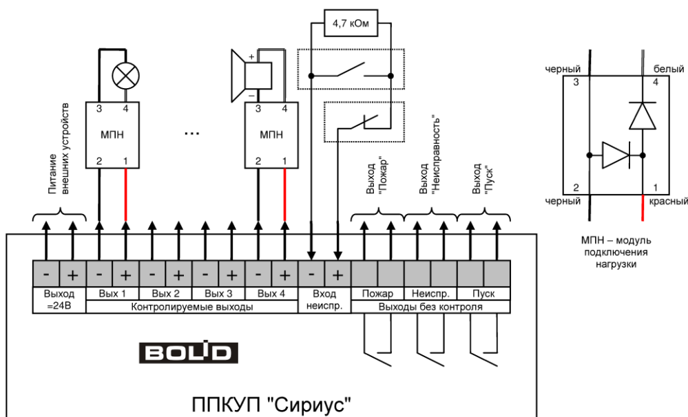
Рисунок 55. Схема подключения дискретных входов и выходов
