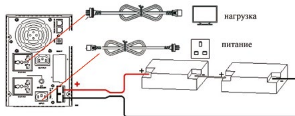
Корпус Tower. 1000 ВА Схема подключения аккумуляторных батарей. Напряжение постоянного тока U=24\text{В} .
