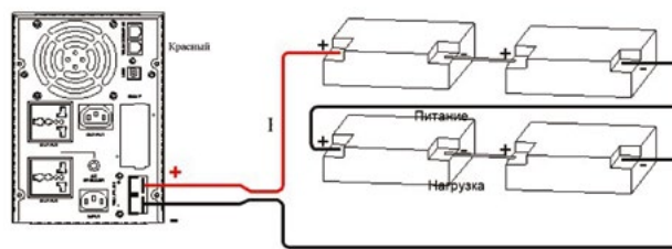
Корпус Tower. Схема подключения аккумуляторных батарей. Напряжение постоянного тока U=48\text{В} .
