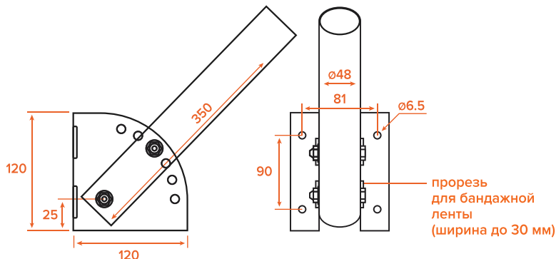
КРОНШТЕЙН НАСТЕННЫЙ/ УНИВЕРСАЛЬНЫЙ K1H-0-035-BM
