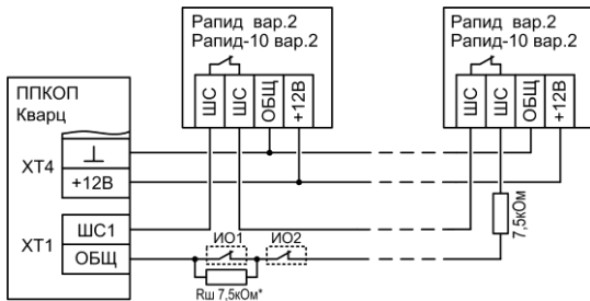
Рис.А8 Схема подключения охранных извещателей Рapid вар.2, Рapid-10 вар.2, ПОЛЮС-2 (ИО1, ИО2)
