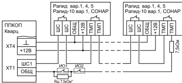
Рис.А9 Схема подключения охранных извещателей Рapid вар.1,4,5, Рapid-10 вар.1, СОНАР, ПОЛЮС-2 (ИО1, ИО2)
