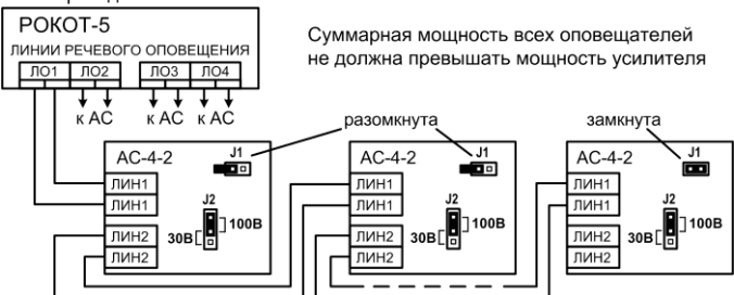
Рис.3 Схема подключения АС к «РОКОТ-5 ПУО-100» и «РОКОТ-5 УМ-100» ВНИМАНИЕ! Для подключения АС к «РОКОТ-5 ПУО-30» и «РОКОТ-5 УМ-30» необходимо установить переключатель J2 на плате АС в положение «30В»
