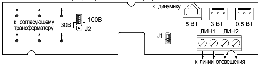
Рис.1 Плата АС
