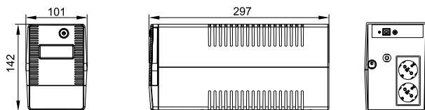
Рисунок 3 – Внешний вид ИБП типа EST-650VA-1-001-S, EST-850VA-1-001-S
