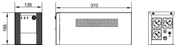
Рисунок 10 – Внешний вид ИБП типа EST-1200VA-1-002-S-L
