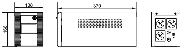
Рисунок 9 – Внешний вид ИБП типа EST-1200VA-1-002-S
