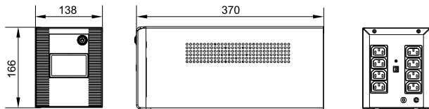
Рисунок 13 – Внешний вид ИБП типа EST-2000VA-1-002
