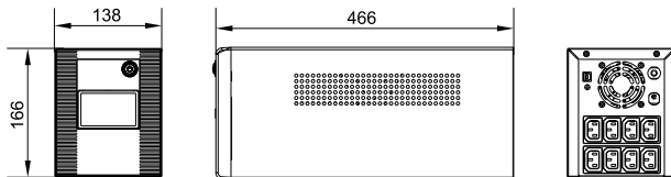
Рисунок 15 – Внешний вид ИБП типа EST-3000VA-1-002
