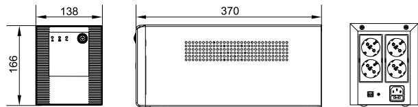
Рисунок 12 – Внешний вид ИБП типа EST-1500VA-1-002-S-L, EST-2000VA-1-002-S-L
