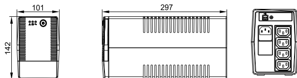
Рисунок 2 – Внешний вид ИБП типа EST-650VA-1-001-L, EST-850VA-1-001-L, EST-1000VA-1-001-L
