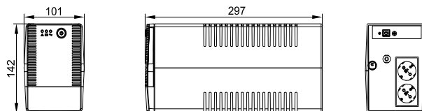
Рисунок 4 – Внешний вид ИБП типа EST-650VA-1-001-S-L, EST-850VA-1-001-S-L
