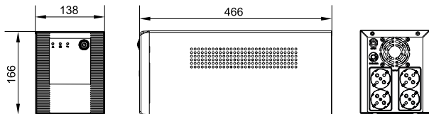
Рисунок 18 – Внешний вид ИБП типа EST-3000VA-1-004-S-L
