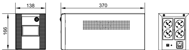
Рисунок 11 – Внешний вид ИБП типа EST-1500VA-1-002-S, EST-2000VA-1-002-S
