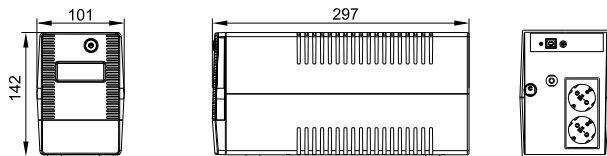
Рисунок 5 – Внешний вид ИБП типа EST-1000VA-1-001-S
