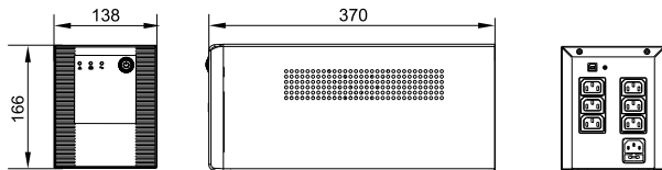
Рисунок 8 – Внешний вид ИБП типа EST-1200VA-1-002-L, EST-1500VA-1-002-L
