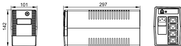
Рисунок 1 – Внешний вид ИБП типа EST-650VA-1-001, EST-850VA-1-001, EST-1000VA-1-001
