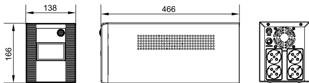
Рисунок 17 – Внешний вид ИБП типа EST-3000VA-1-004-S
