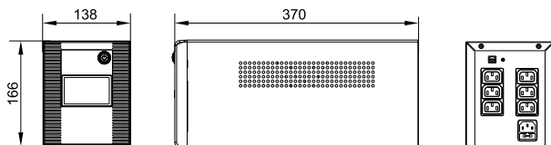
Рисунок 7 – Внешний вид ИБП типа EST-1200VA-1-002, EST-1500VA-1-002
