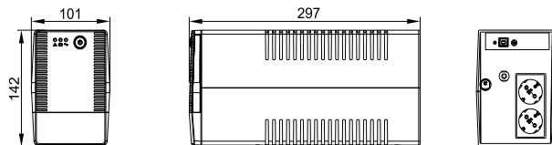
Рисунок 6 – Внешний вид ИБП типа EST-1000VA-1-001-S-L
