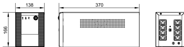
Рисунок 14 – Внешний вид ИБП типа EST-2000VA-1-002-L
