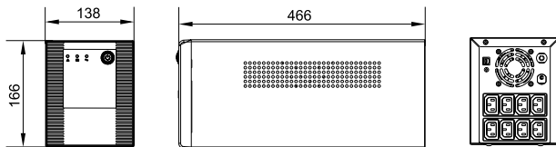
Рисунок 16 – Внешний вид ИБП типа EST-3000VA-1-004-L
