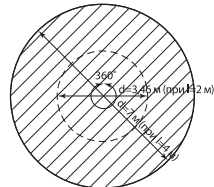
Рисунок 3. Зона обнаружения датчиками движения ДДП-01, ДДП-02, ДДП-03, ДДП-05
